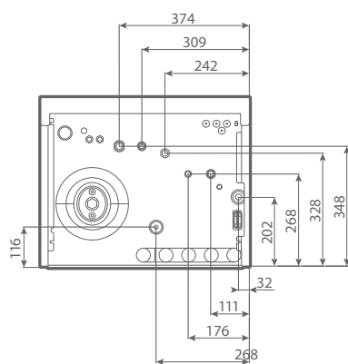
Vista inferiore
