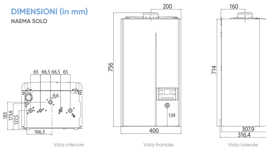
Vista inferiore
