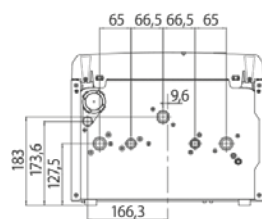
Vista inferiore
