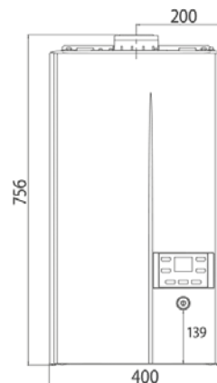
Vista frontale
