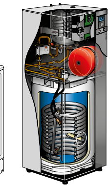
Alfea Excellia Duo A.I. con opzione integrazione caldaia e kit 2 circuiti
