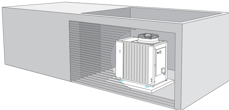
Installation en semi extérieur avec champ libre sur le dessus
