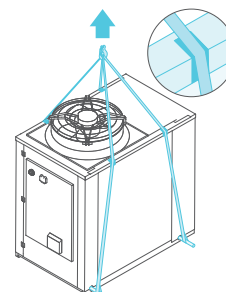
Levage avec système d'élingues
