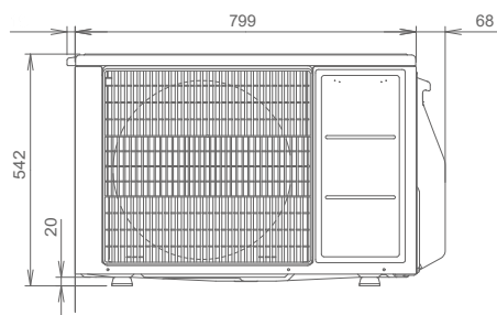
Vooraanzicht
