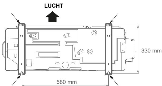
Onderaanzicht
