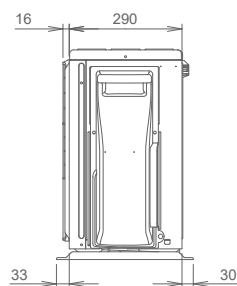
Linksaanzicht
