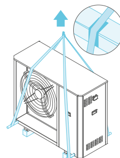
Levage avec système d'élingues
