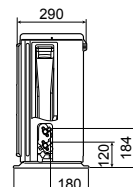
Vue de côté
