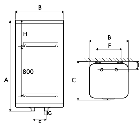
STEATITE CUBE 150
